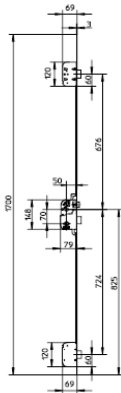
Serrure 3 pts Pènes rectangulaires Longueur 1700 mm
