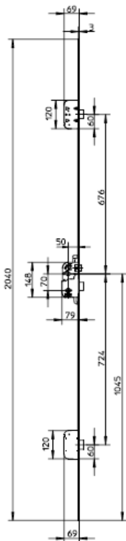
Serrure 3 pts Pènes rectangulaires Longueur 2040 mm
